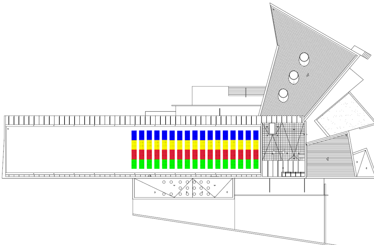
Figura 8. Disposición de los paneles fotovoltaicos sobre la cubierta.
