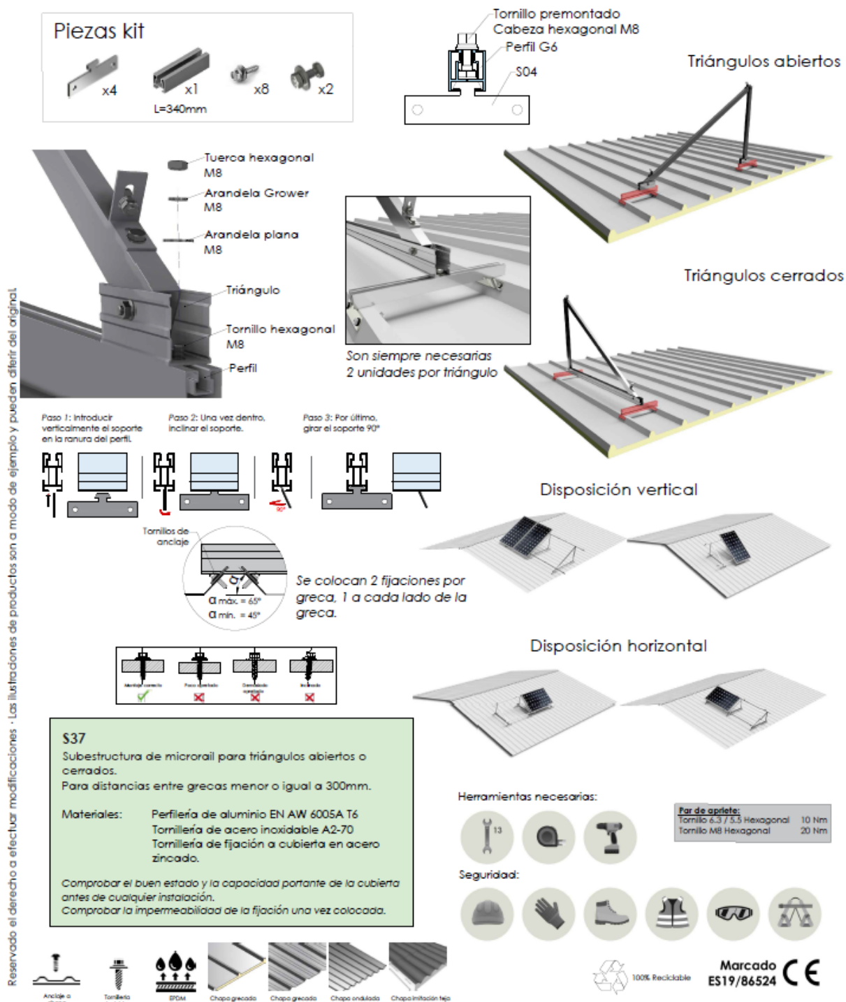
Figura 7. Fijación estructura metálica sobre la cubierta
