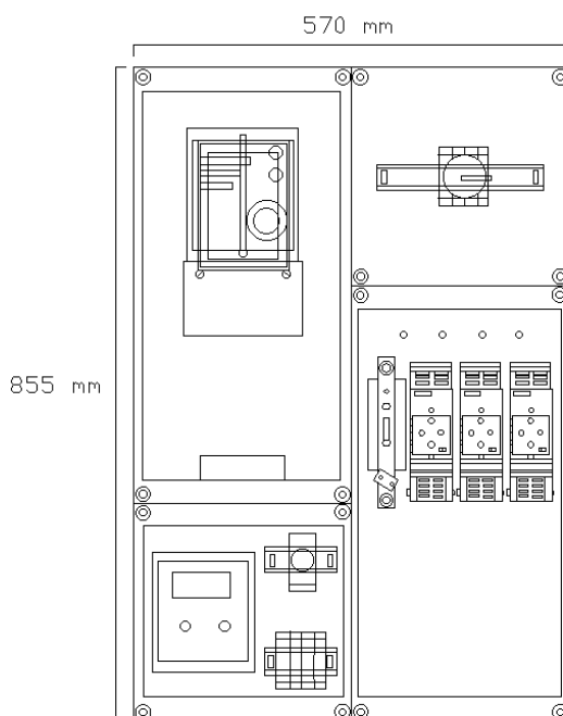
Figura 11. TMF-1.
