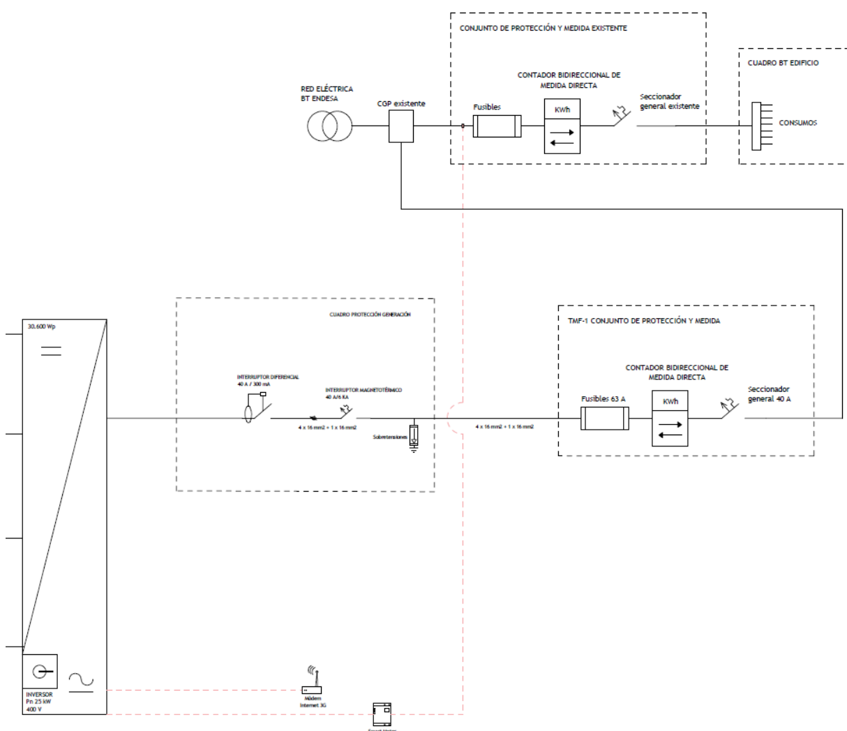
Figura 5. Esquema de conexión del lado de corriente alterna inversor
