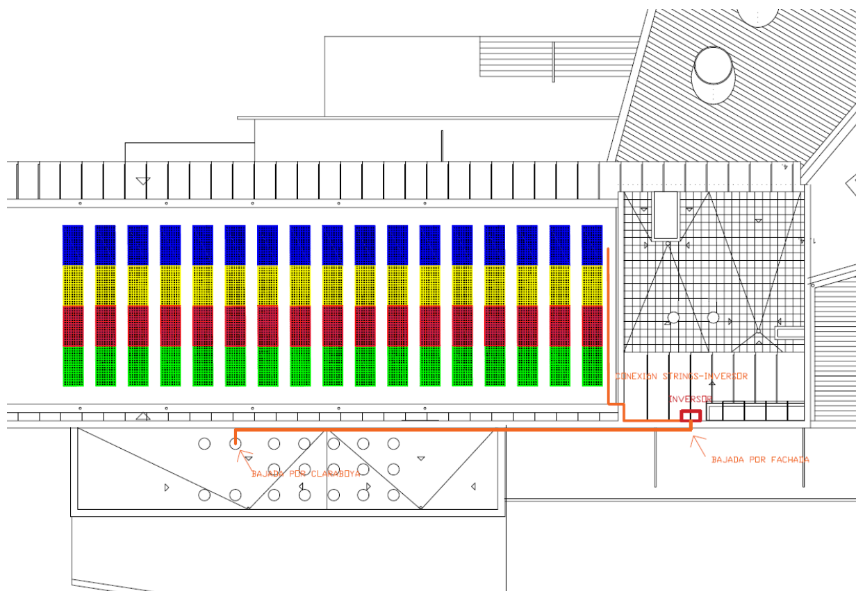
Figura 9. Distribución strings-cajas de protección-inversor.
