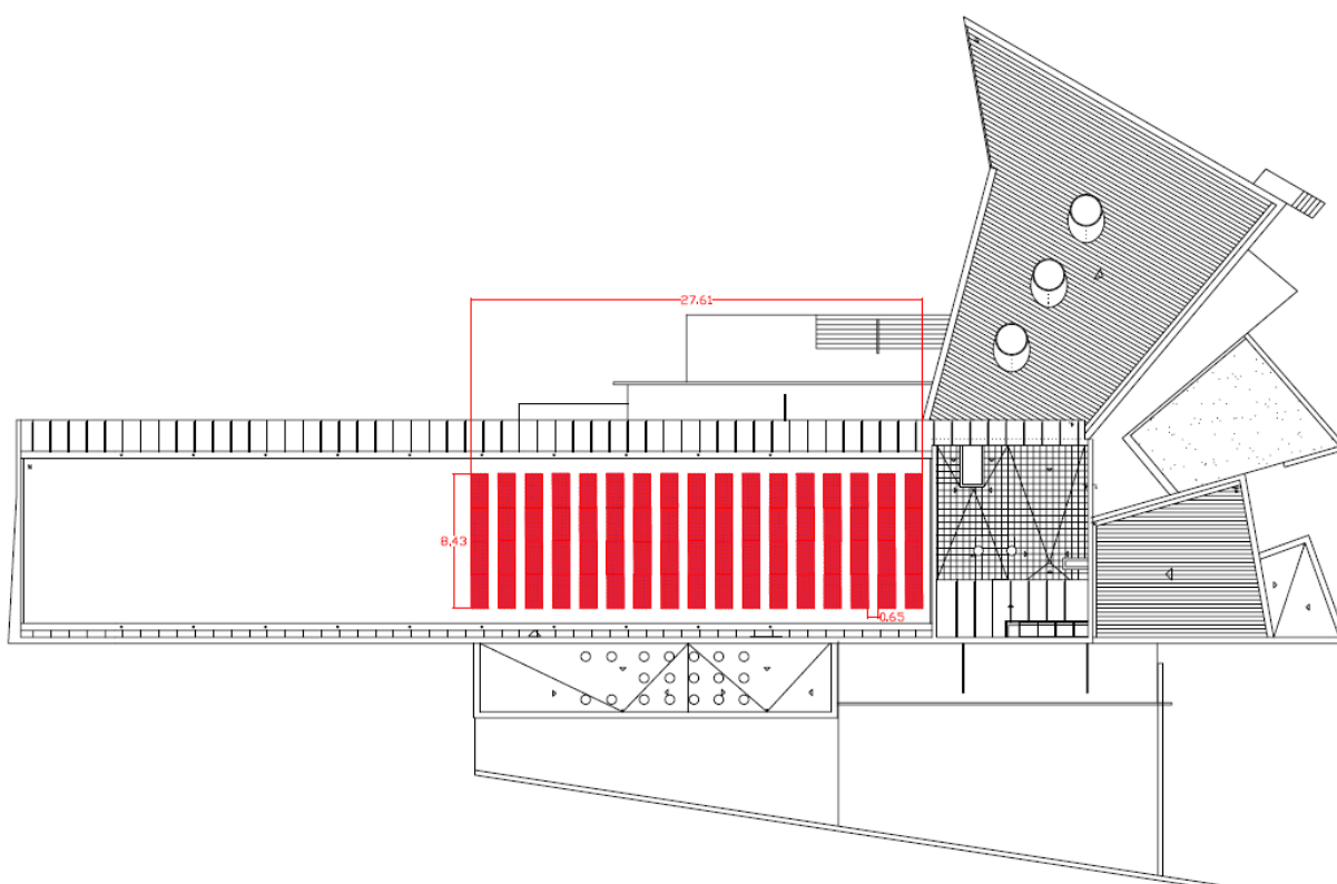
Figura 2. Disposición física de la zona habilitada donde irán ubicadas las placas fotovoltaicas.
