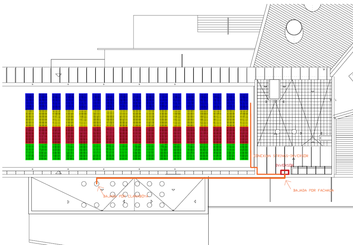
Figura 10. Conexión inversor hasta punto de red.
