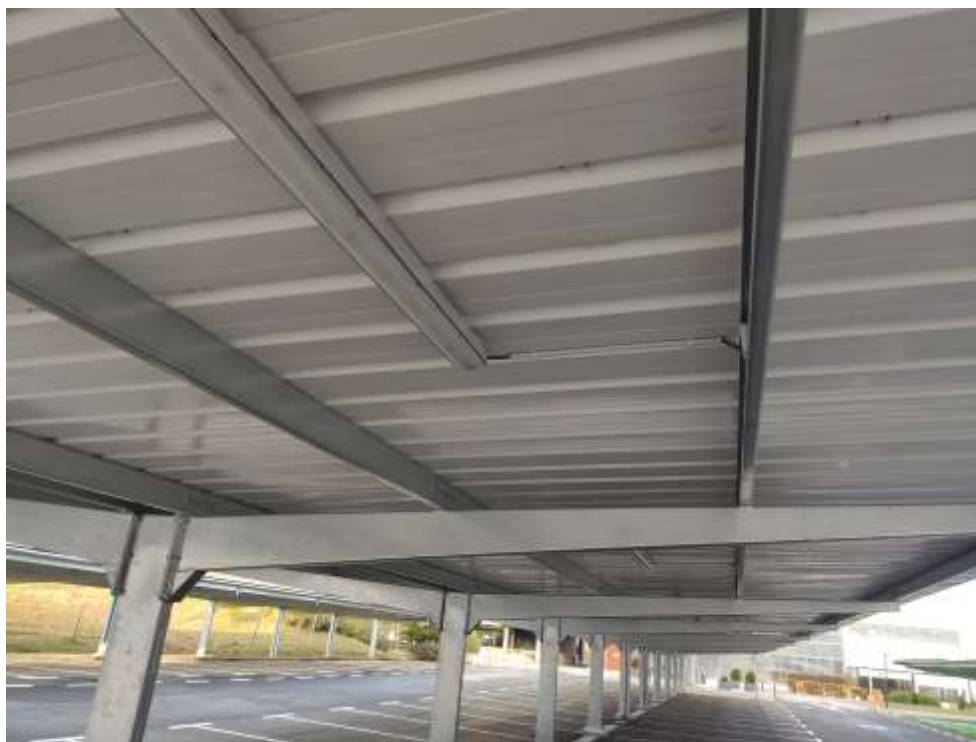
Vista des de sota d'una mènsula doble
