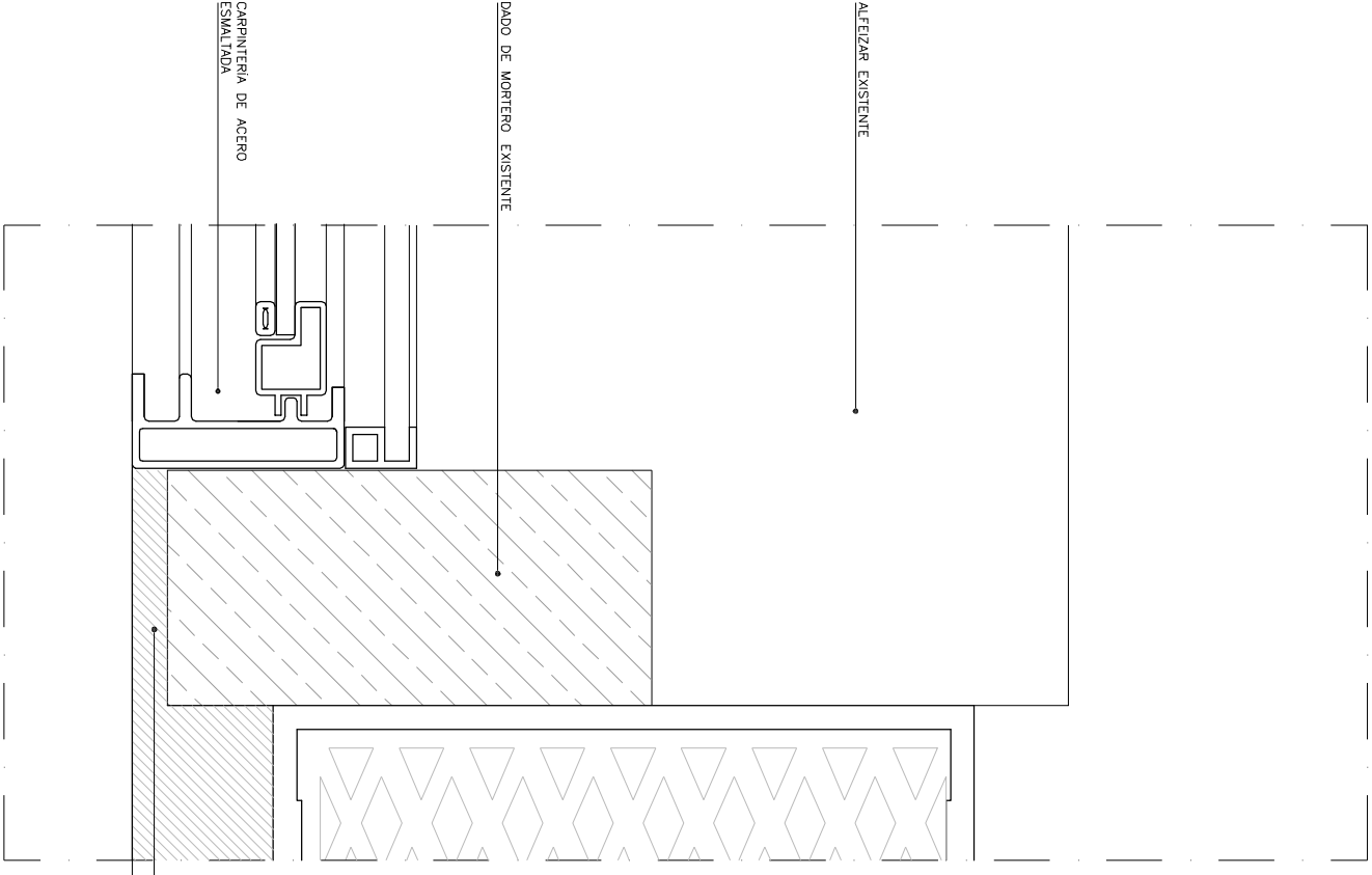
JB-DETALLE JAMBA TIPO ESTADO ACTUAL ESCALA 1:2
