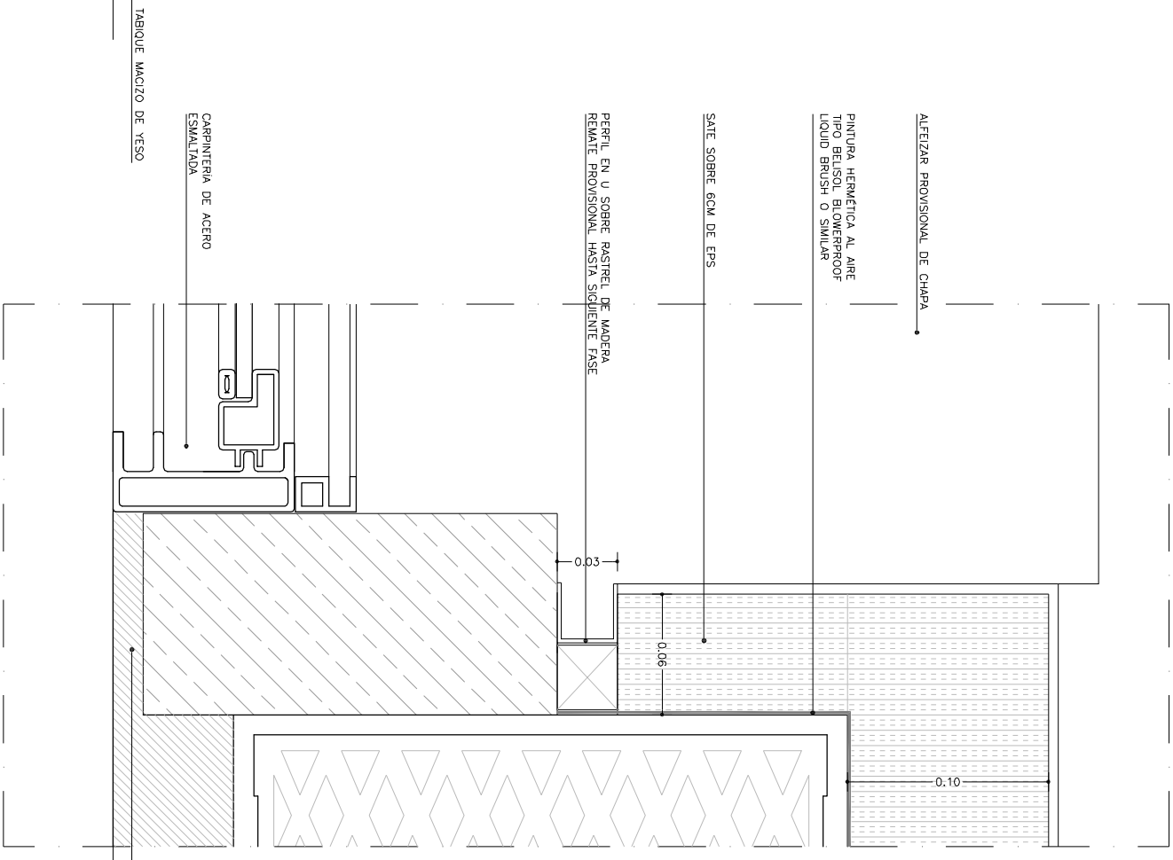
JB-DETALLE JAMBA PRIMERA FASE JAMBA VENTANA CON PANEL 6CM ESCALA 1:2
